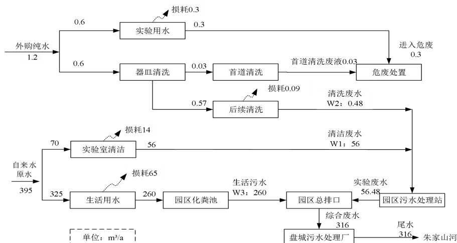
图 4-2 项目水平衡图
