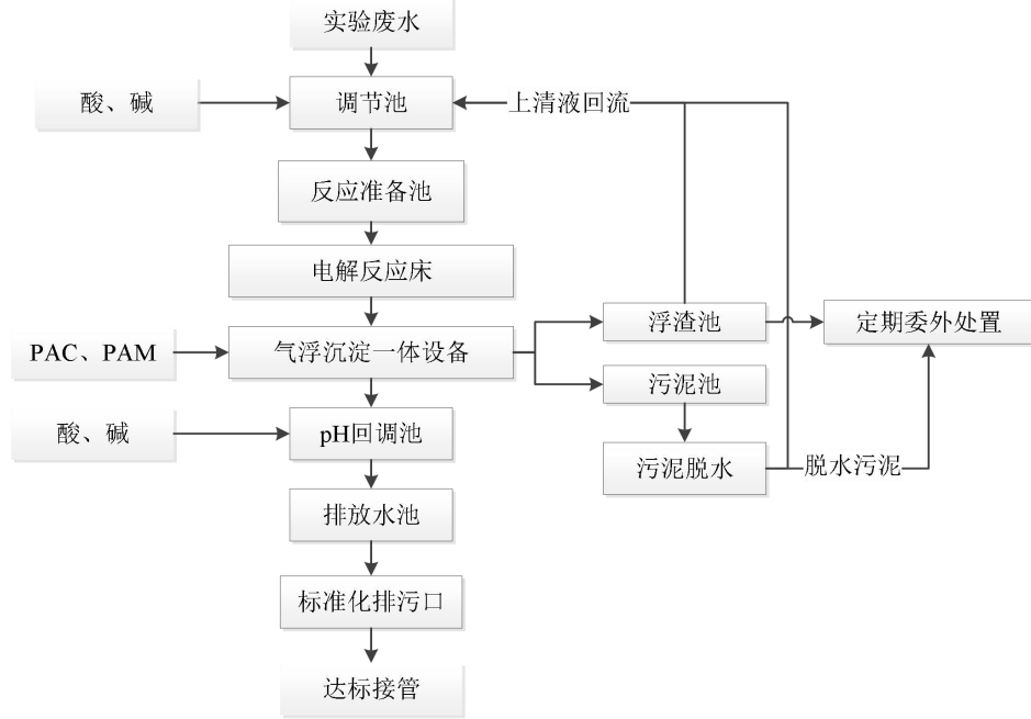
图 4-3 鼎业百泰生物大楼污水处理设施工艺流程示意图
