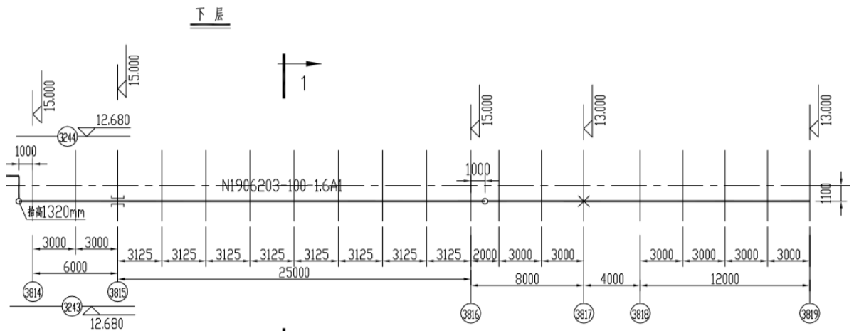
图 1-1 氮气管线柱 3814~柱 3819 段断面示意图
