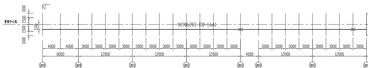
图 1-2 氮气管线柱 3819~3826 段断面示意图
