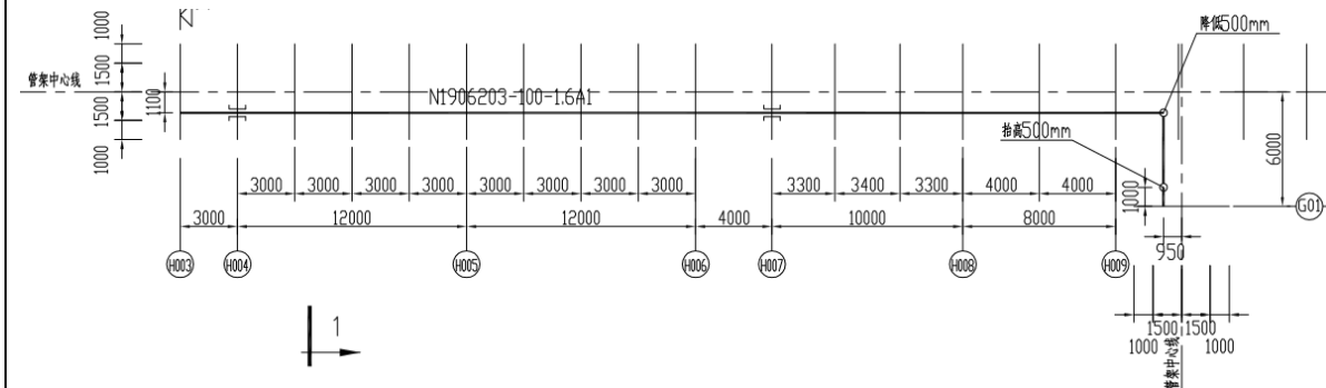
图 1-6 氮气管线柱 H003~H009 段断面示意图
