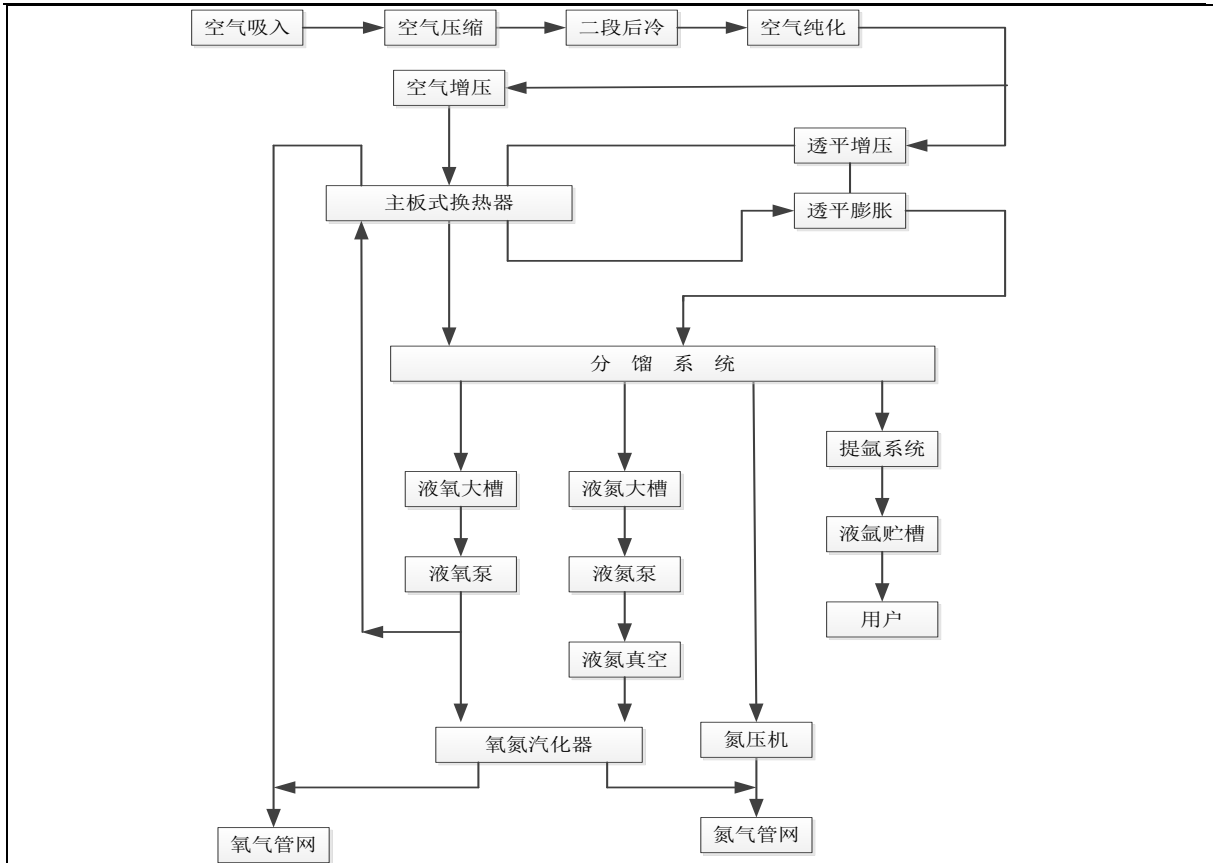
图 1-11 C/D 套空分工艺流程图
