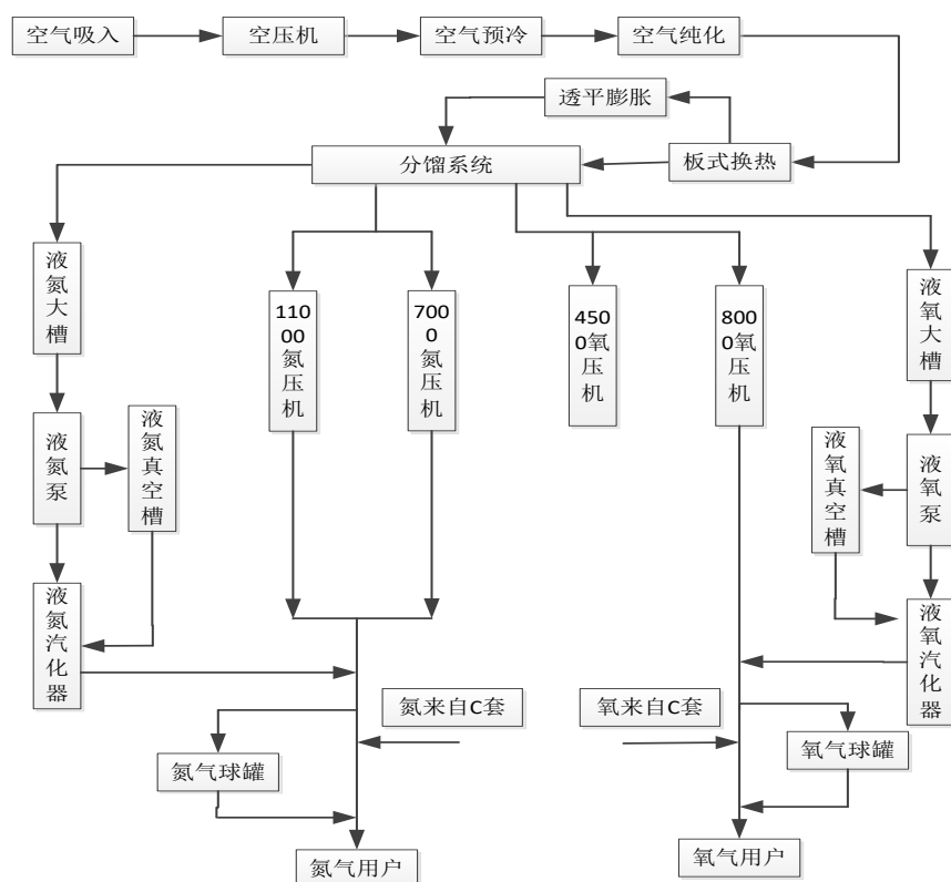
图 1-10 A/B 套空分工艺流程图
